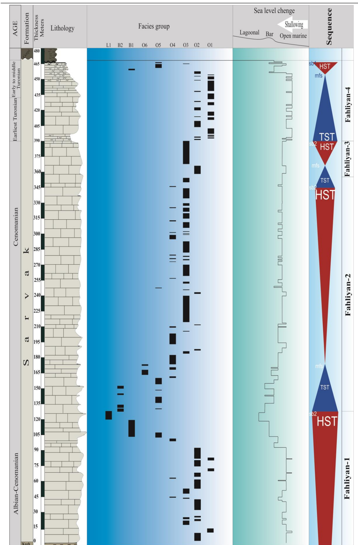
شکل ۴- ستون ریز رخساره و چینه نگاری سکانسی سازند سروک در برش ناقدیس فهلیان.
